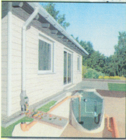
①雨水利用 雨水利用タンクにゴミがはいら ないようにする。
